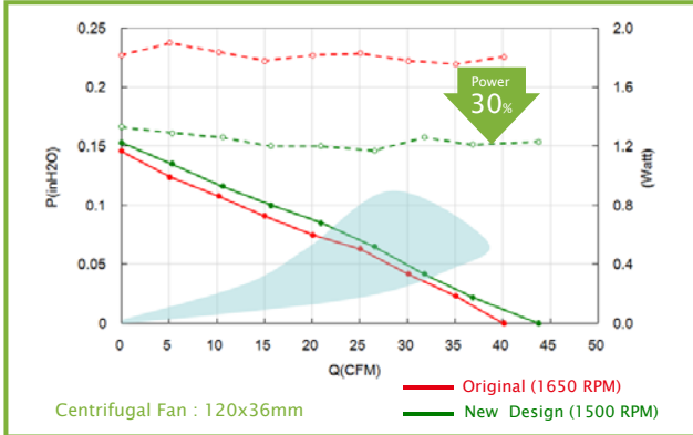
Centrifugal Fan : 120x36mm
