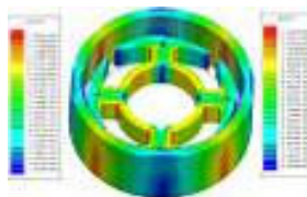
馬達磁路模擬分析
