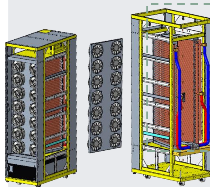
AALC 氣冷輔助液冷散熱櫃 散熱冷排 (60~80kW)
